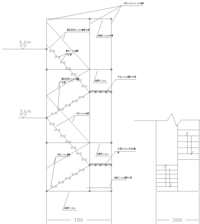
云海湾别墅群入户临时钢管楼梯示意图
